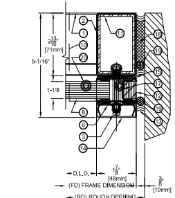
F JAMB DETAIL - RIGHT SCALE: N.T.S.
