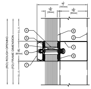
B SILL DETAIL SCALE: N.T.S.
