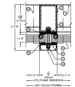
E VERTICAL MULLION SCALE: N.T.S.
