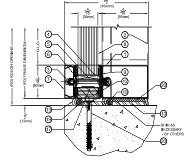
B SILL DETAIL SCALE: N.T.S.
