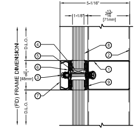
C HORIZ. MULLION DETAIL SCALE: N.T.S.
