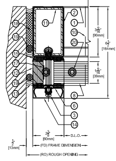
D JAMB DETAIL - LEFT SCALE: N.T.S.
