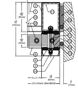
F JAMB DETAIL - RIGHT SCALE: N.T.S.
