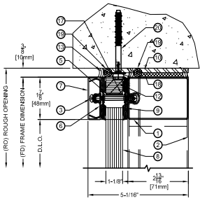
A HEAD DETAIL SCALE: N.T.S.
