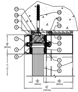
A HEAD DETAIL SCALE: N.T.S.
